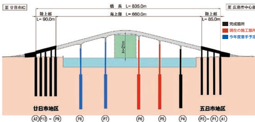
(はつかいち大橋の工事進捗状況 (一般図))
